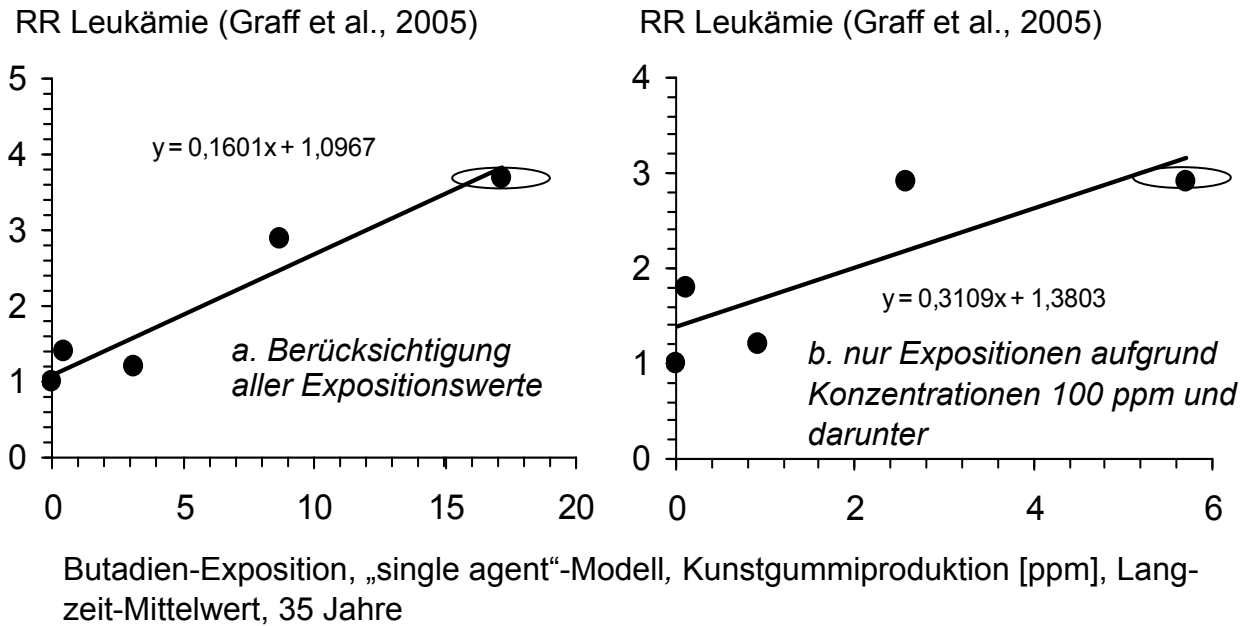
Abb. 1: Relative Raten (RR) der Leukämiemortalität in Abhängigkeit von der Butadien-Exposition, umgerechnet auf mittlere Konzentration über 35 Jahre, nach Daten der Studie von Graff et al. (2005). Durch Ellipsen ist angedeutet, dass die Angabe eines mittleren Expositionswerts für die oberste - nach oben offene - Kategorie mit Unsicherheiten behaftet ist.
