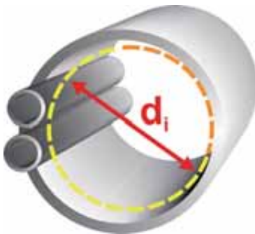
Abbildung 3: Bestimmung des lichten Durchmessers d_i (Lichtmaß)
