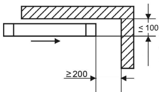
Abb. 2: Vermeiden von Quetschgefahren zum Schutz des Kopfbereiches
